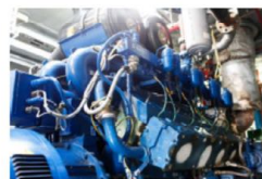
716 kWel BHKW
